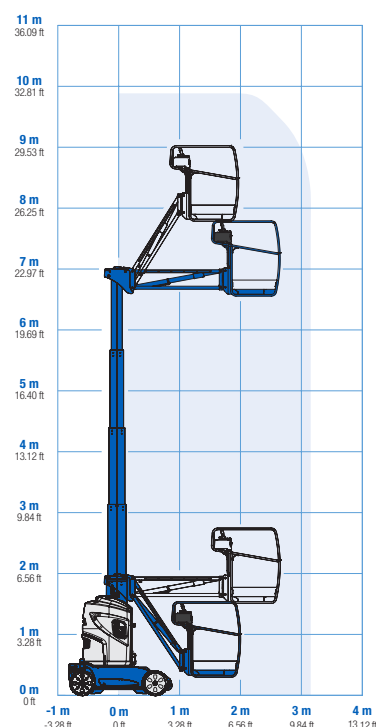
Courbe de travail GR-26 J
